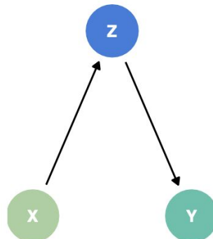
(3) Mediator
